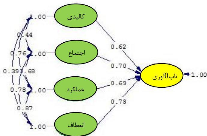
تصویر ۵. مدل ساختاری (MES) ضریب پیوستگی پیرسون و ارتباط بین شاخص‌ها
