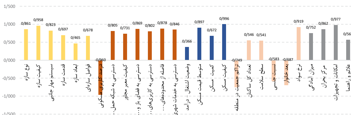
تصویر ۴. میزان بار عاملی متغیرها (بر اساس داده‌های جدول ۹)
