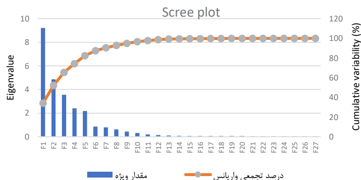
تصویر ۳. نمودار سنگریزه مقدار ویژه مؤلفه‌های استخراج شده (حاصل از روش PCA)
